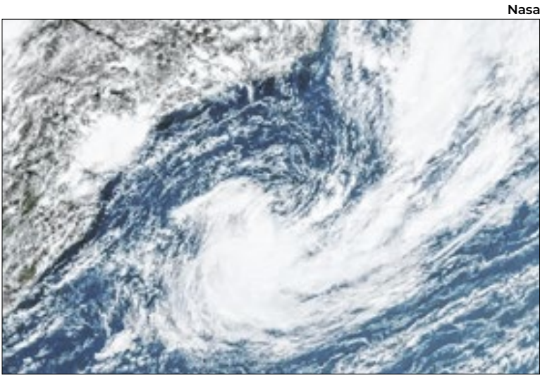
Instabilidades são devido a ciclone extratropical
