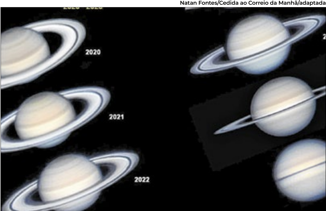
A sequência mostra como os anéis desaparecem conforme a inclinação de Saturno
