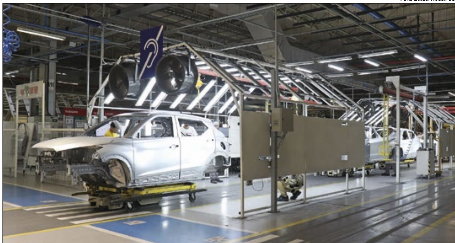
Fábrica de Resende faz todas as etapas de montagem de um veículo
